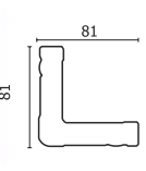
Панель B10, B15, B20, B25, B30-126
