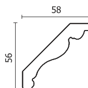
DD Карниз A1080-WG (58x56)
