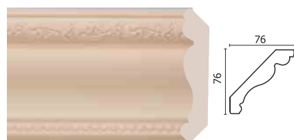
Карниз 154-62
