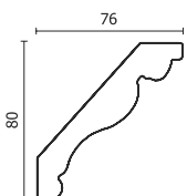
DD Карниз A1011-WG (76x80)
