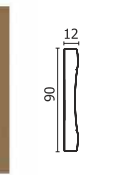
Молдинг 151-127
