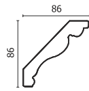
Молдинг 158-1
