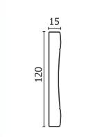
Молдинг 147-127
