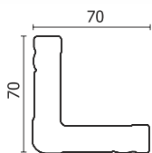
DD Уголок C1070-WG (70x70)
